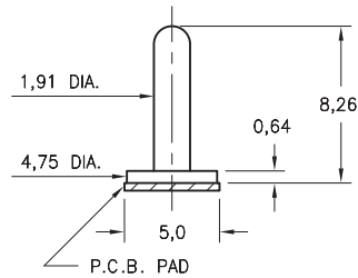
P.C.B. PAD
