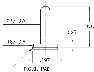
P.C.B. PAD
